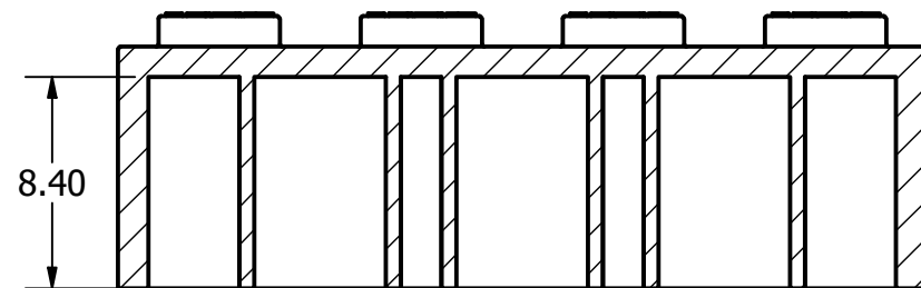
SECTION A-A
